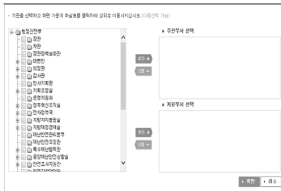
< 화면2 - 다중처리부서지정 >
