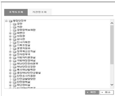
< 화면1 - 처리부서지정 >
